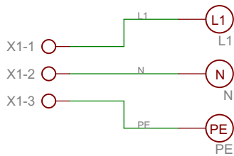
Steckerbelegung Anschlussklemmen Netzspannung
