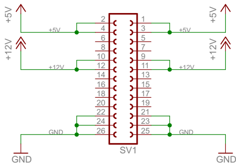
Pinbelegung Buchsenleiste Niederspannung
