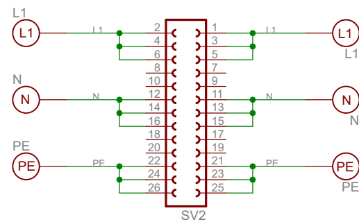
Pinbelegung Buchsenleiste Hochspannung
